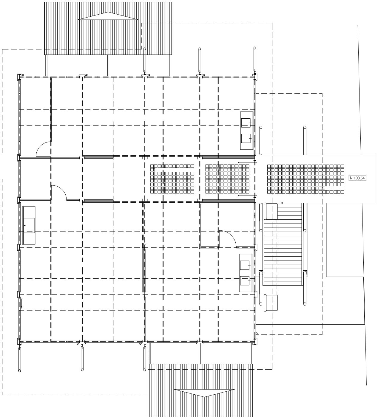
PLANTA DE DISTRIBUCIÓN · SEGUNDO PISO · TALLERES DE ARTE
