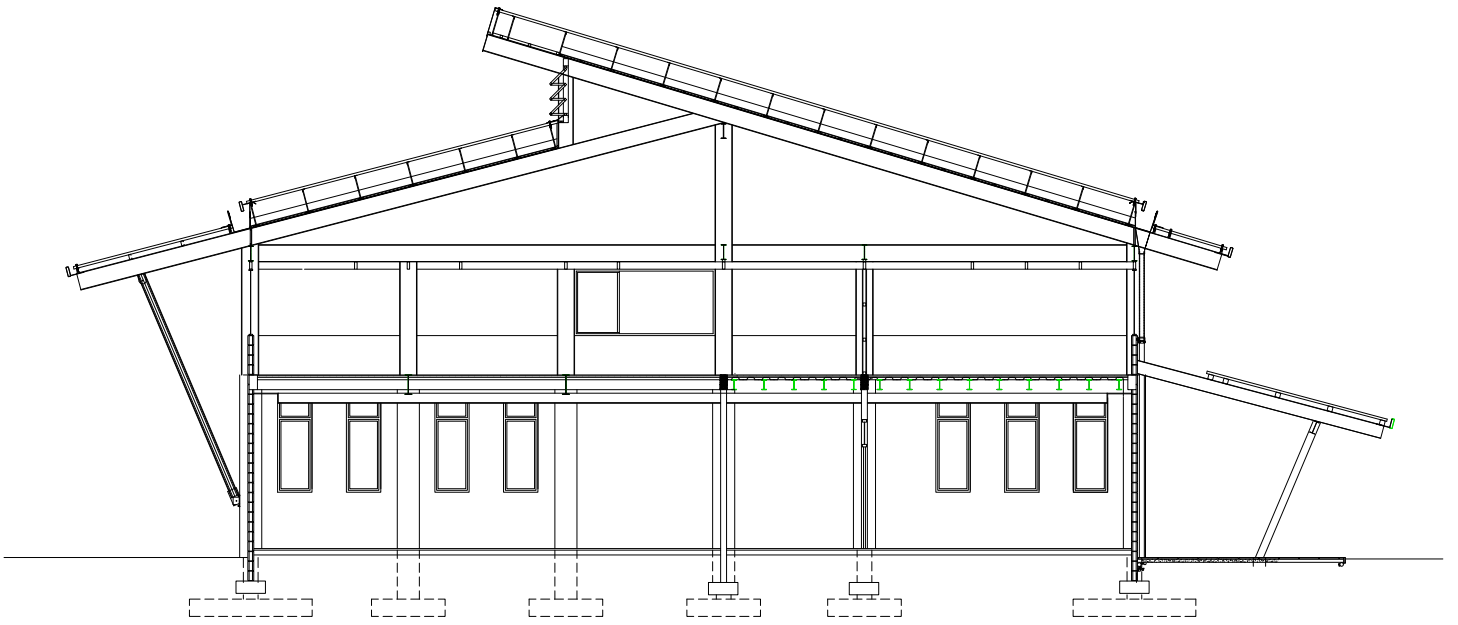
SECCIÓN TRANSVERSAL
