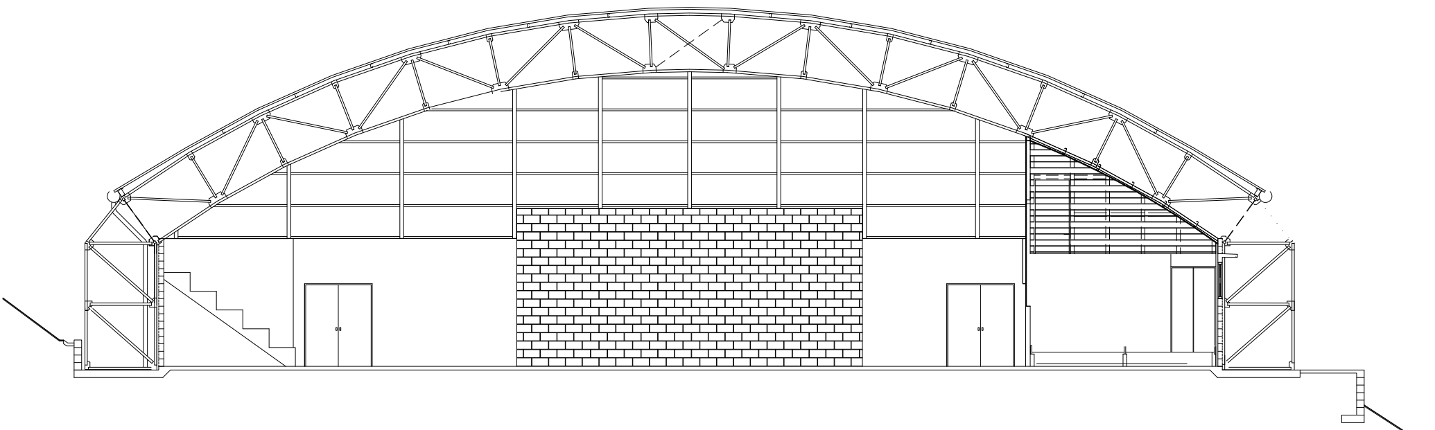
SECCIÓN TRANSVERSAL
