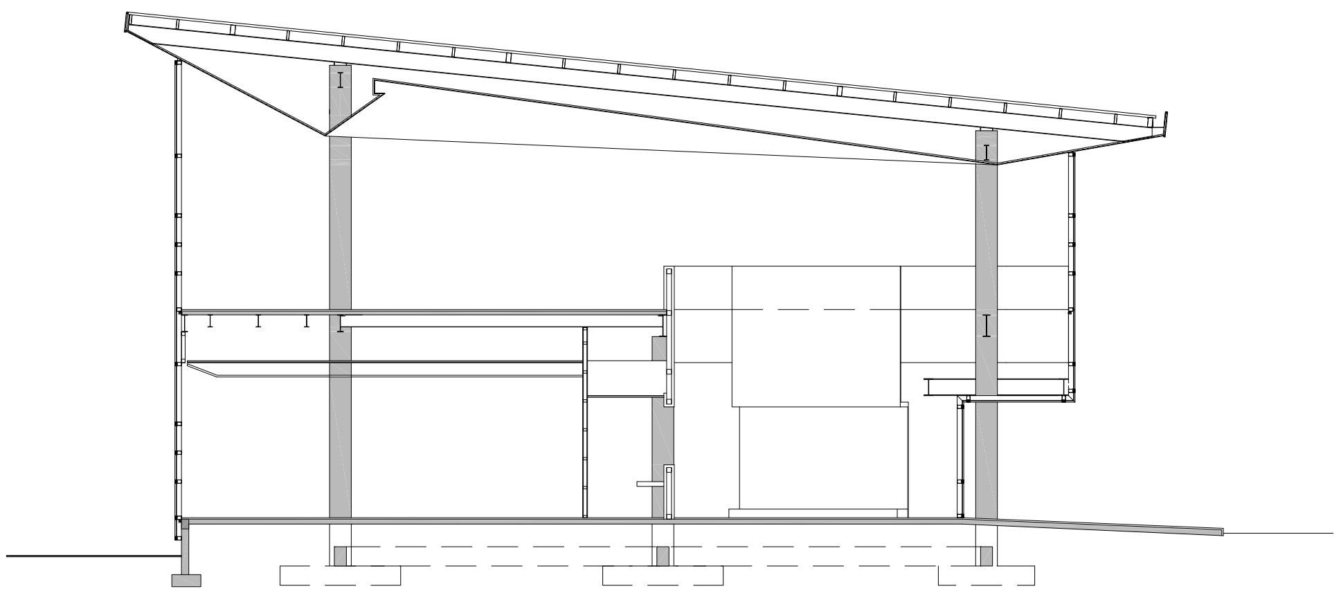
SECCIÓN TRANSVERSAL
