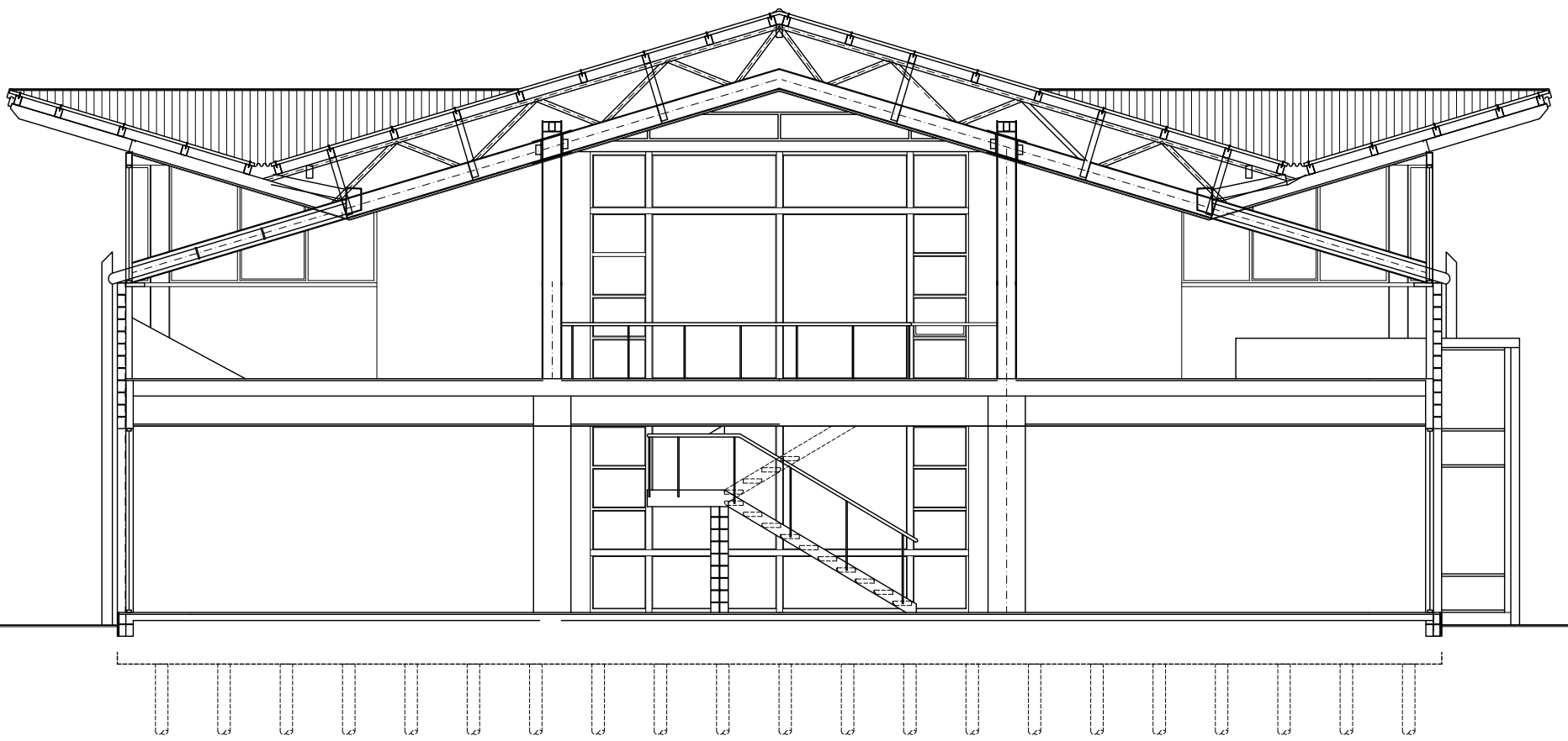
SECCIÓN TRANSVERSAL
